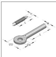
Śruba z łbem oczkowym
