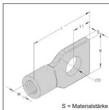
Łącznik Duplo
